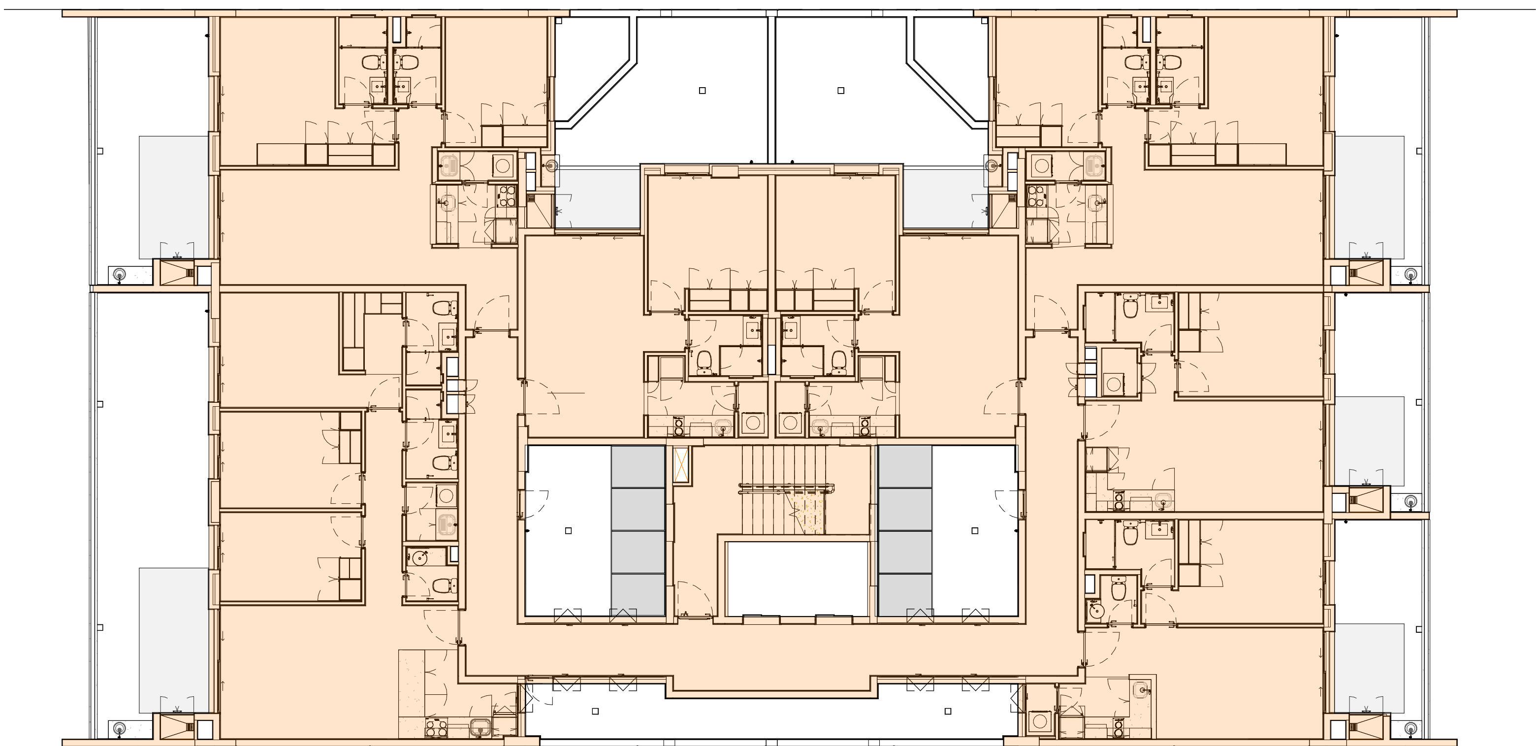
3 Nivel 1 - Departamentos 1:100
