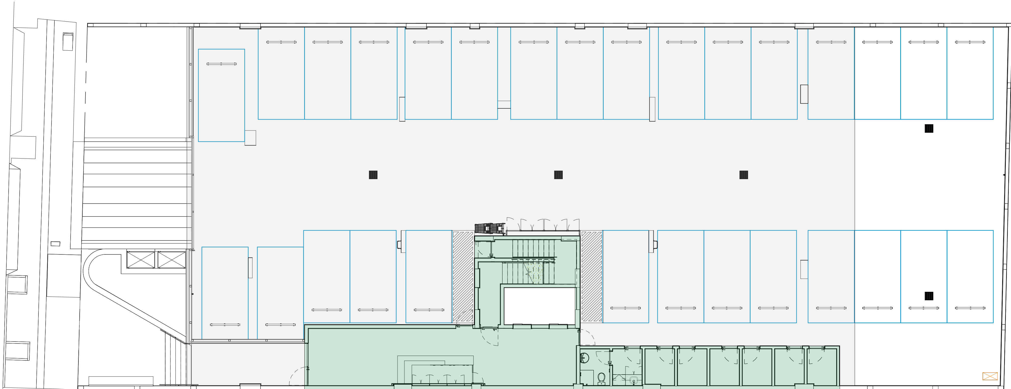
2 Planta Baja - Estacionamiento 1:100
