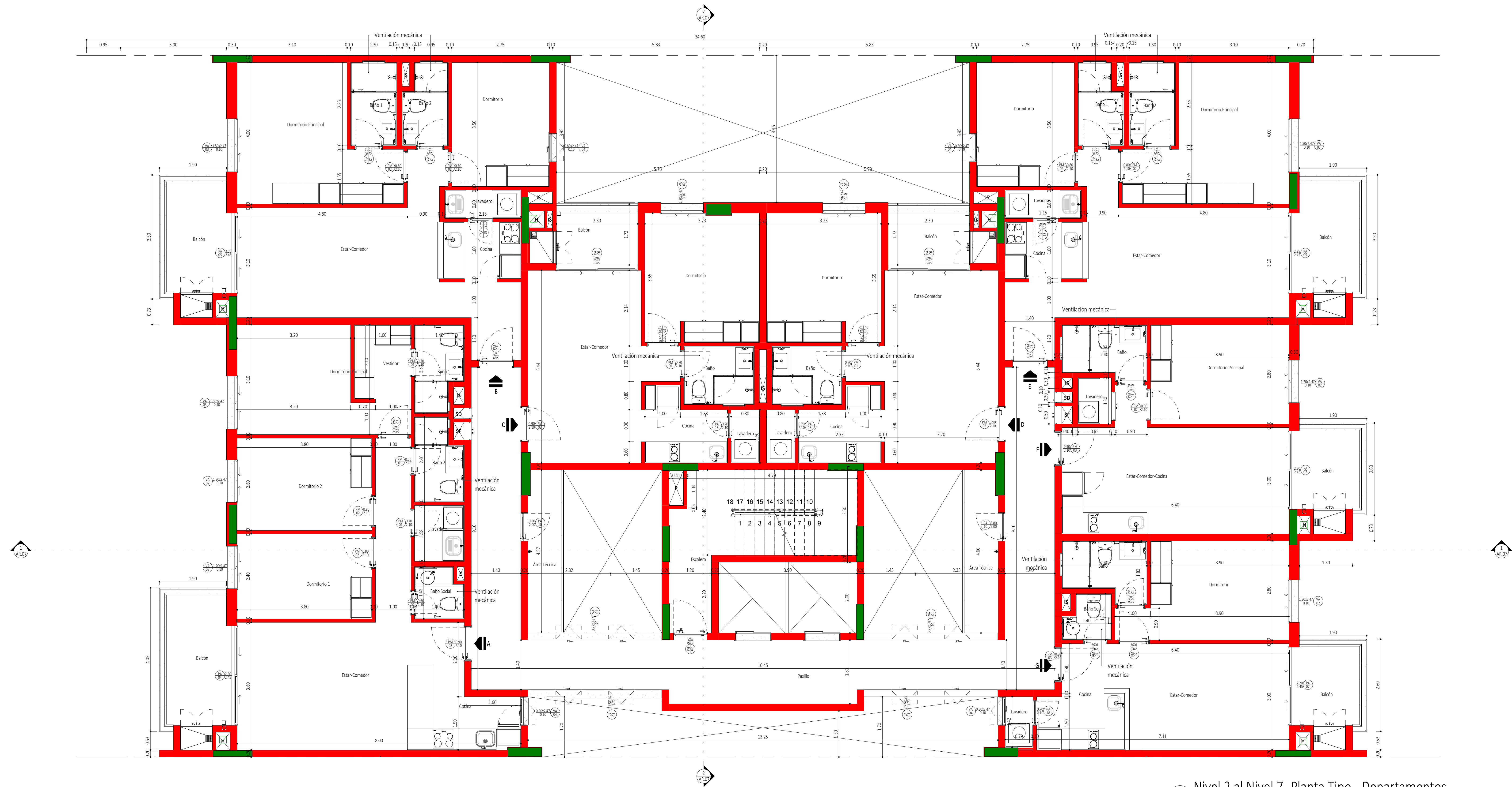
1 Nivel 2 al Nivel 7- Planta Tipo - Departamentos 1:50
