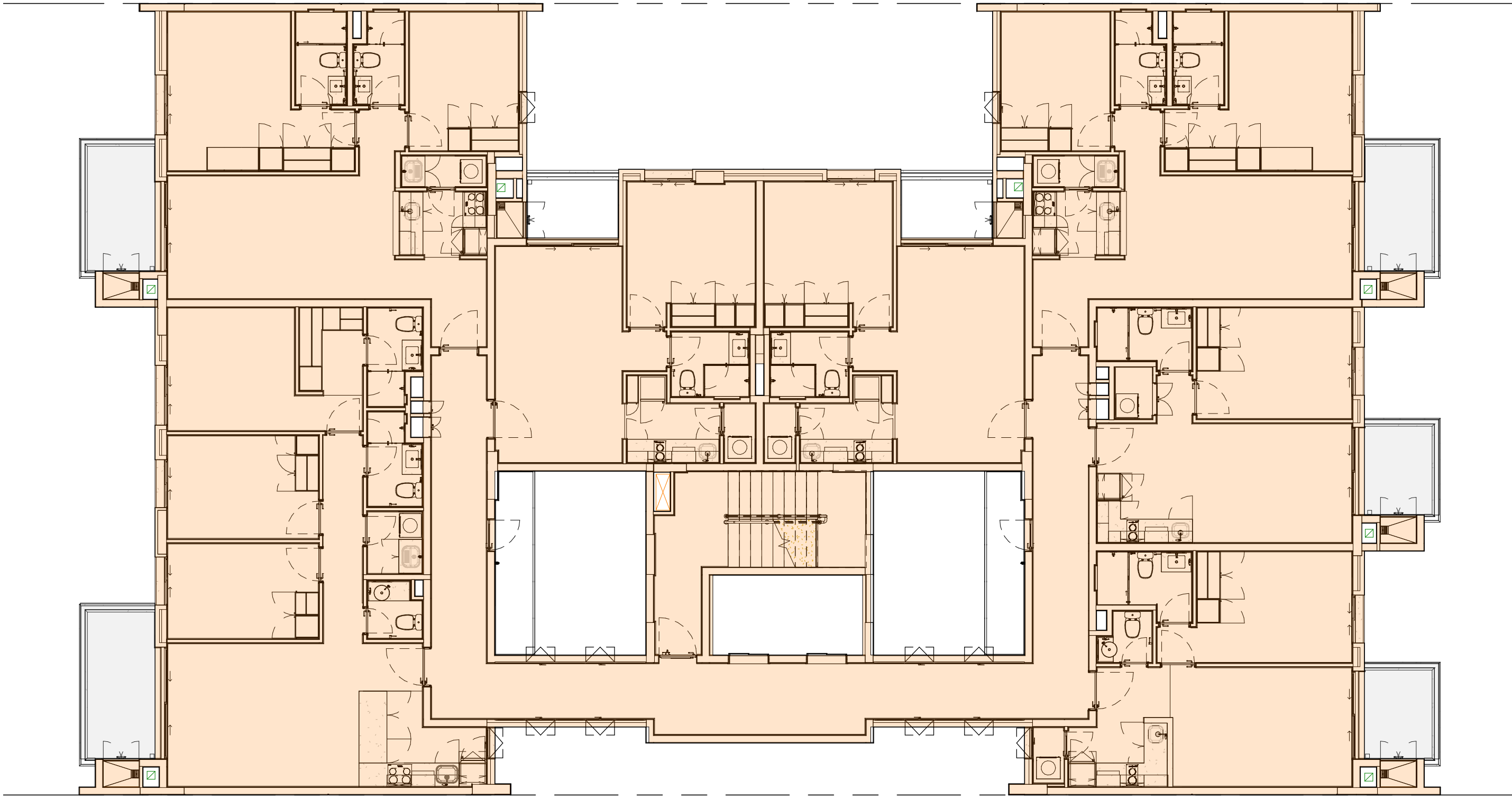
4 Nivel 2 al Nivel 7- Planta Tipo - Departamentos 1:100
