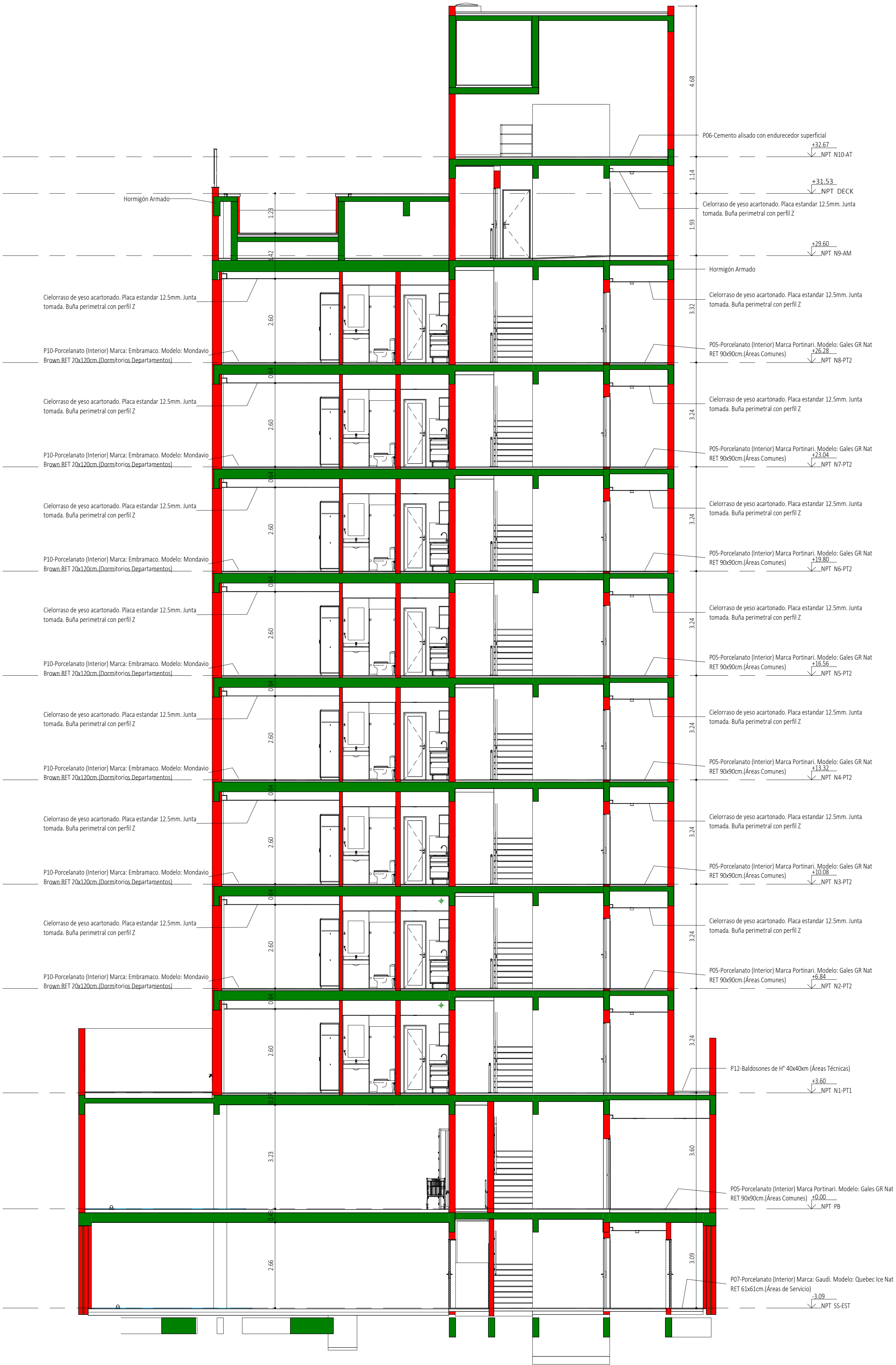
2 Corte 2 1:75
