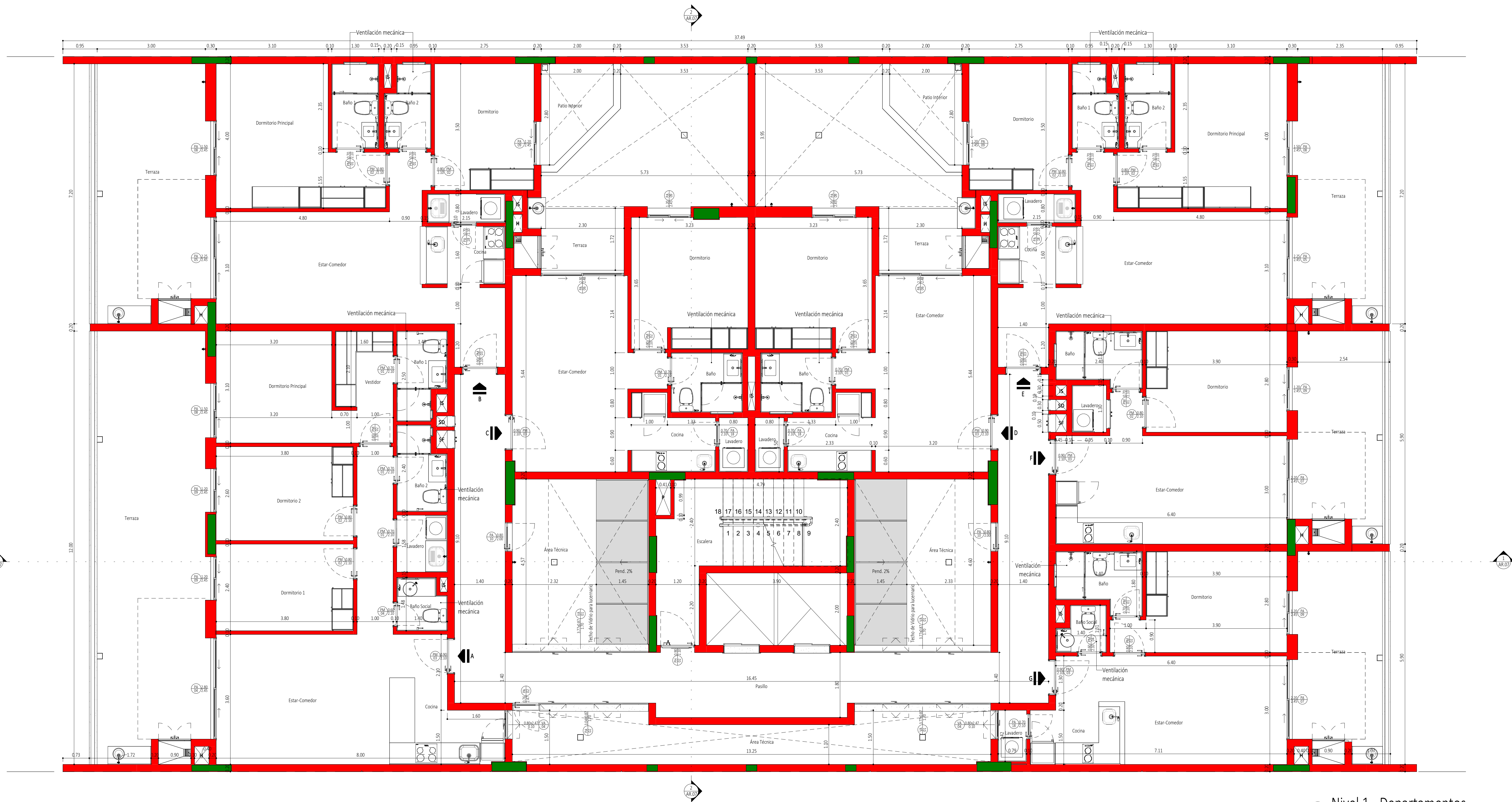
1 Nivel 1 - Departamentos 1:50
